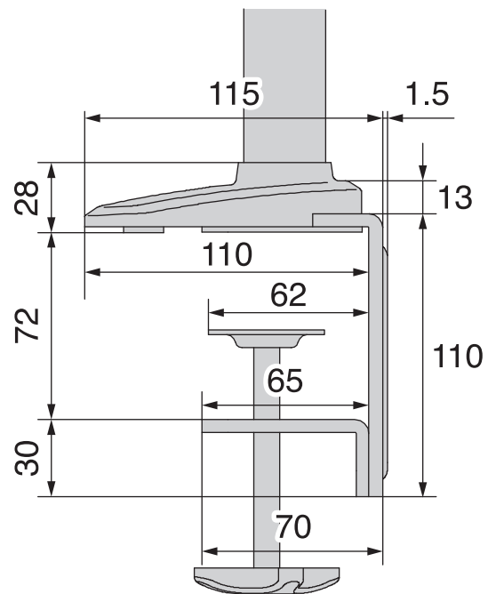
【側面図1】
