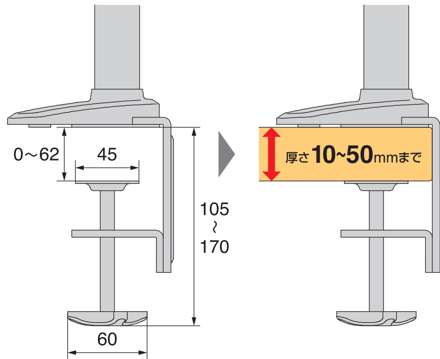
【側面図2】
