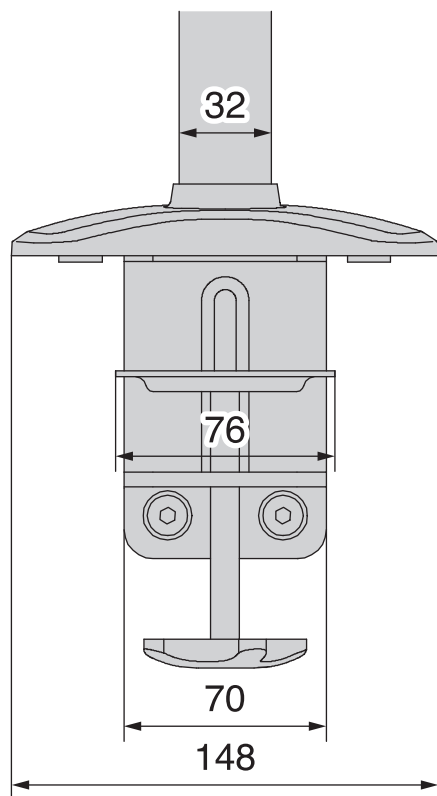
【正面図】
